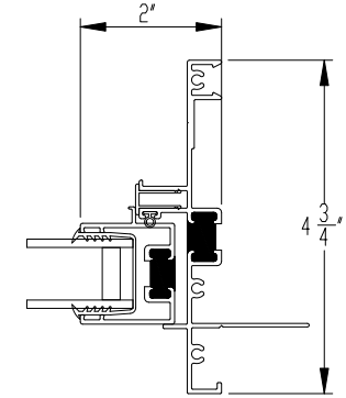
8 FIXED JAMB
