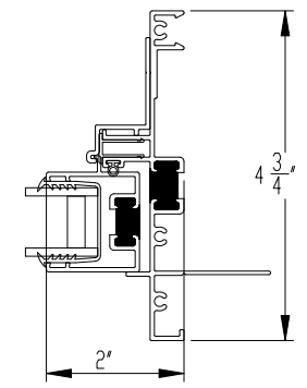
4 FIXED JAMB
