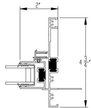
8 FIXED JAMB
